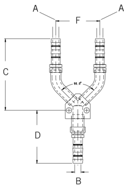
Y Splicer
